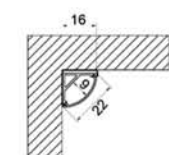
EAAP59 Dimension
