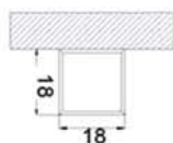
EAAP28 Dimension
