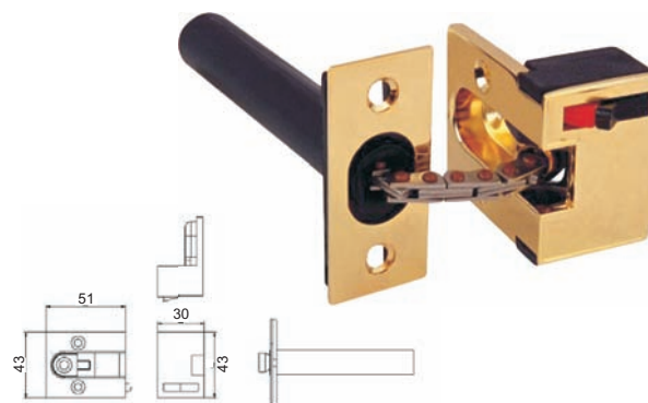
DGS201 - SS Concealed Door Chain
